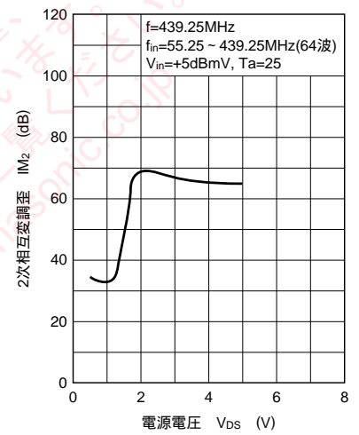
IM_2 - V_{DS}
