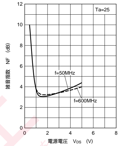
NF - V_{DS}
