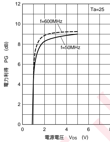
PG - V_{DS}
