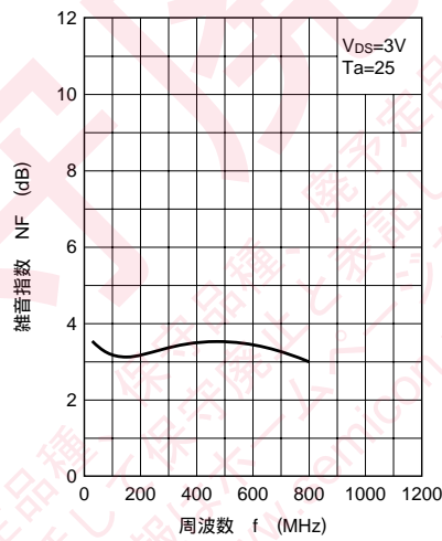
NF - f
