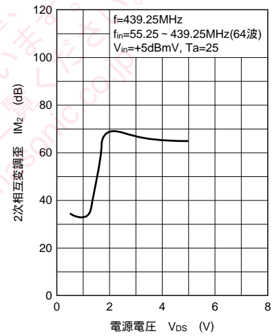
IM_2 - V_{DS}
